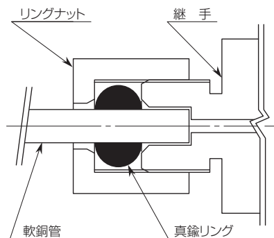
図-1 給水軟銅管の接続
