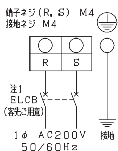
(図7) 電源端子台の接続
