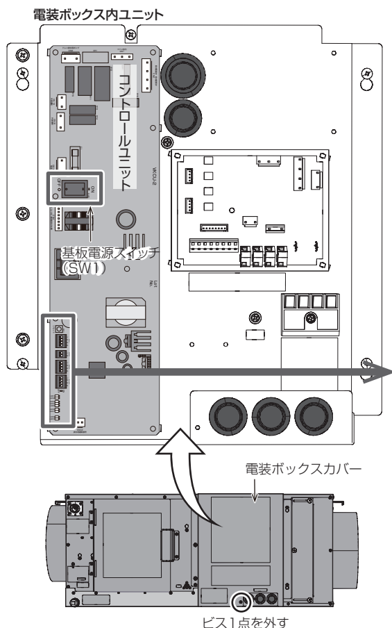
図-3 コントロールユニット外観略図とLED表示内容
