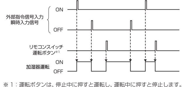
図-9 瞬時入力信号動作タイミングチャート (ヒューミディスタット ON 時)
