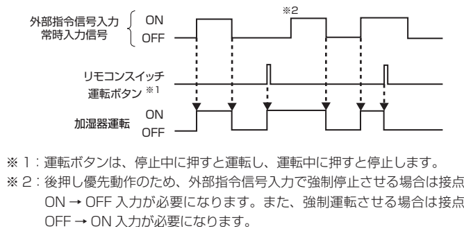
図-8 常時入力信号動作タイミングチャート (ヒューミディスタット ON 時)
