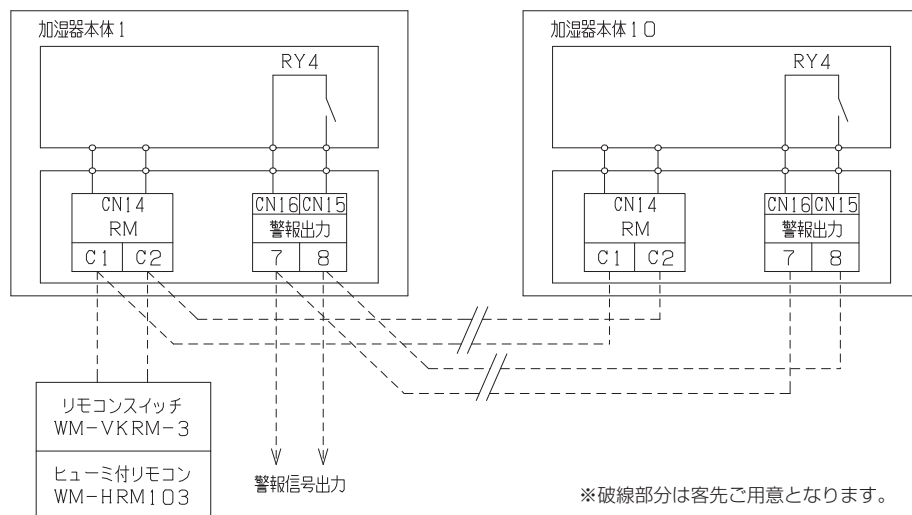
図-6 グループ毎に「警報信号」を出力させる場合の結線参考図
