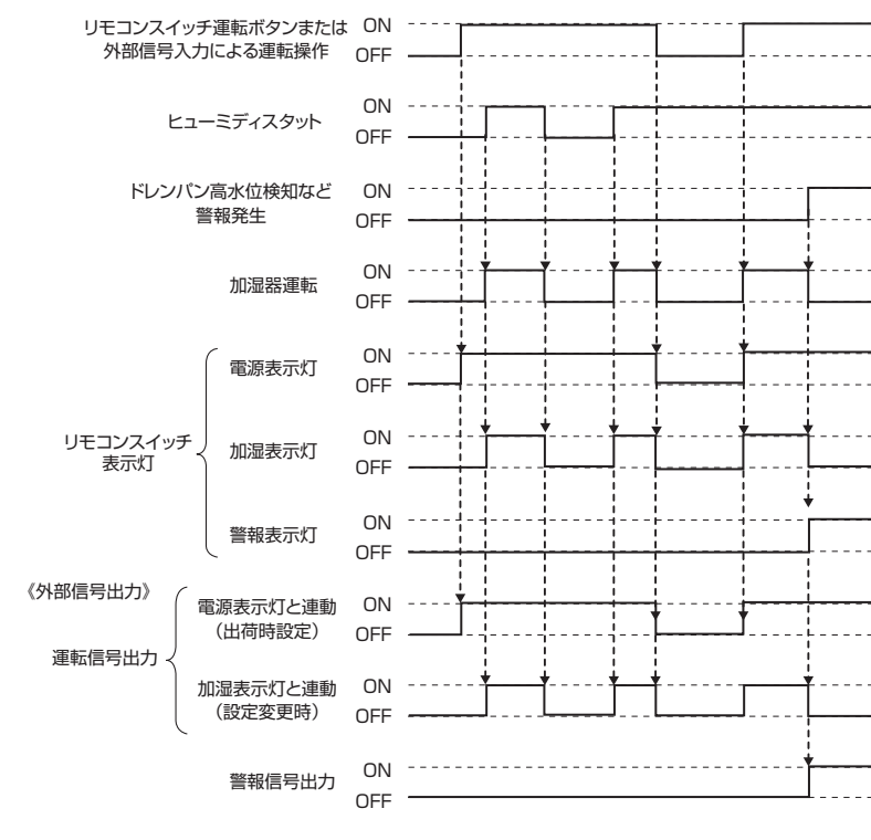
図-10 運転信号出力タイミングチャート
