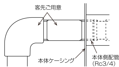
図-5 配管接続
