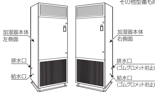
図-4 加湿器本体左右側面 イラストは VFC5000 を表していますが、その他型番も同様です。
