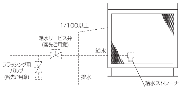
図-3 配管接続 イラストは VFC5000 を表していますが、その他型番も同様です。
