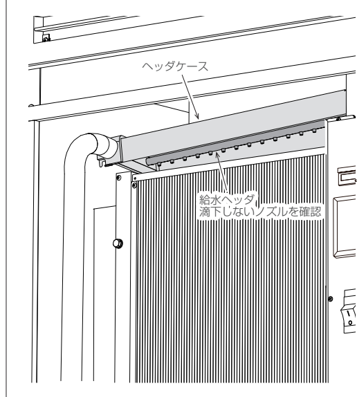
図-34 ノズルからの滴下状態確認
