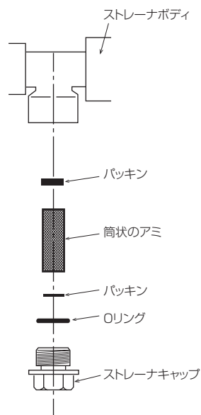
図-22 ストレーナ分解図
