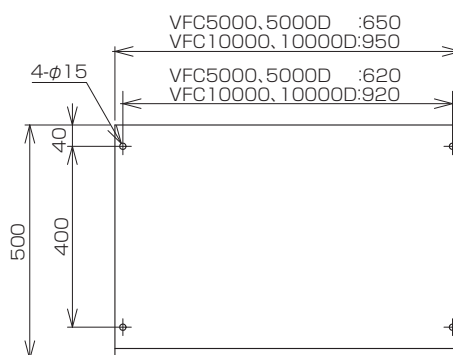
図-2 取付寸法
