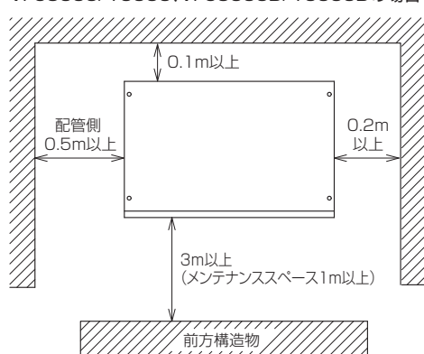
図-1 本体周囲スペース
