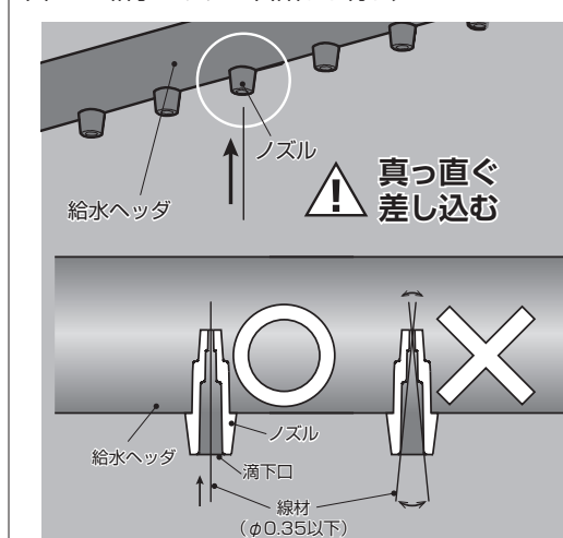
図-35 給水ヘッダの目詰まり除去
