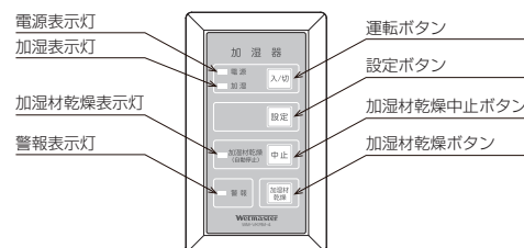
図-36 操作スイッチ詳細
