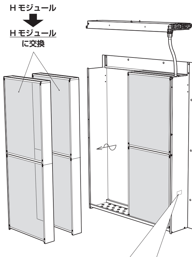
加湿材取付位置図
