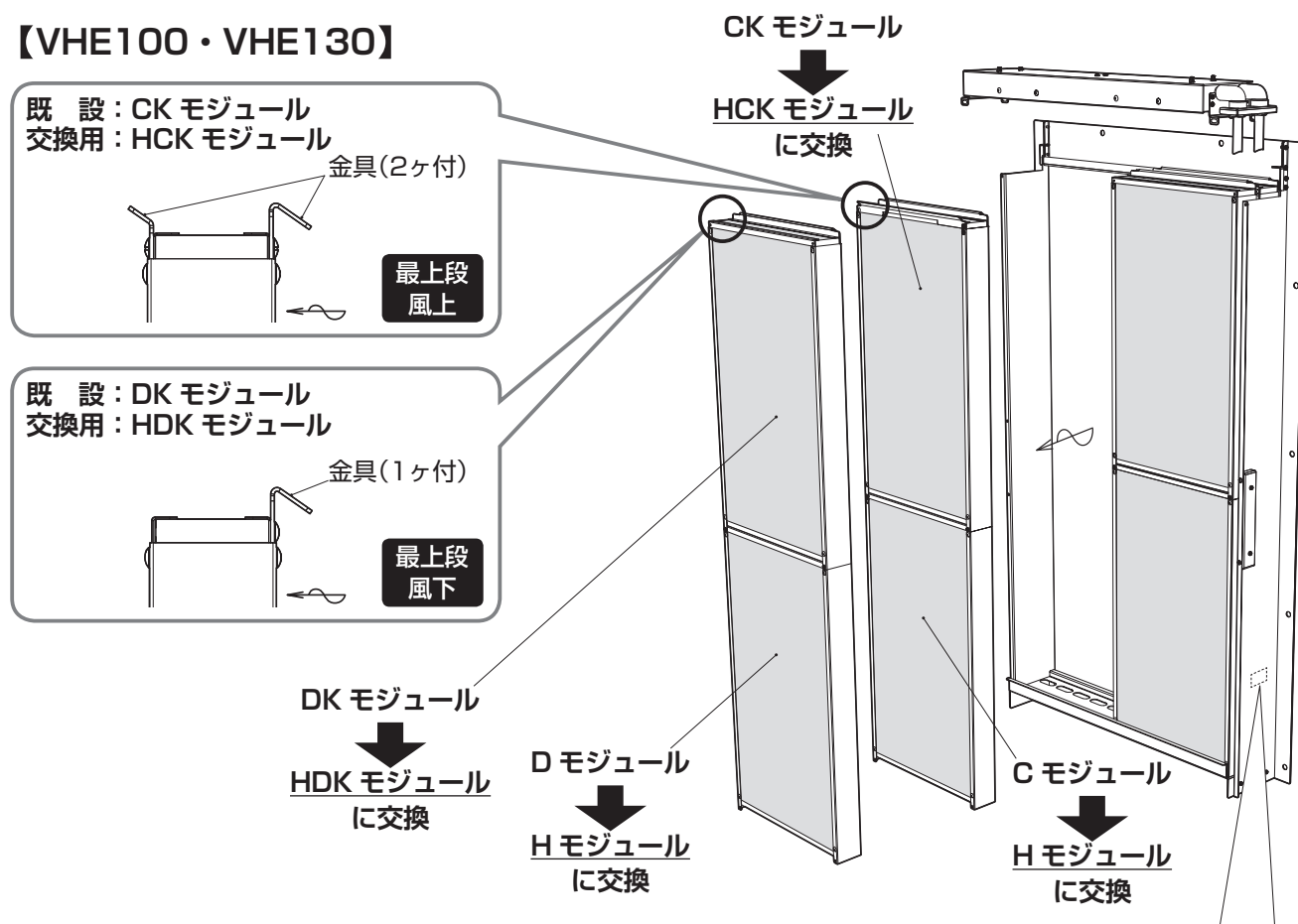
加湿材取付位置図
