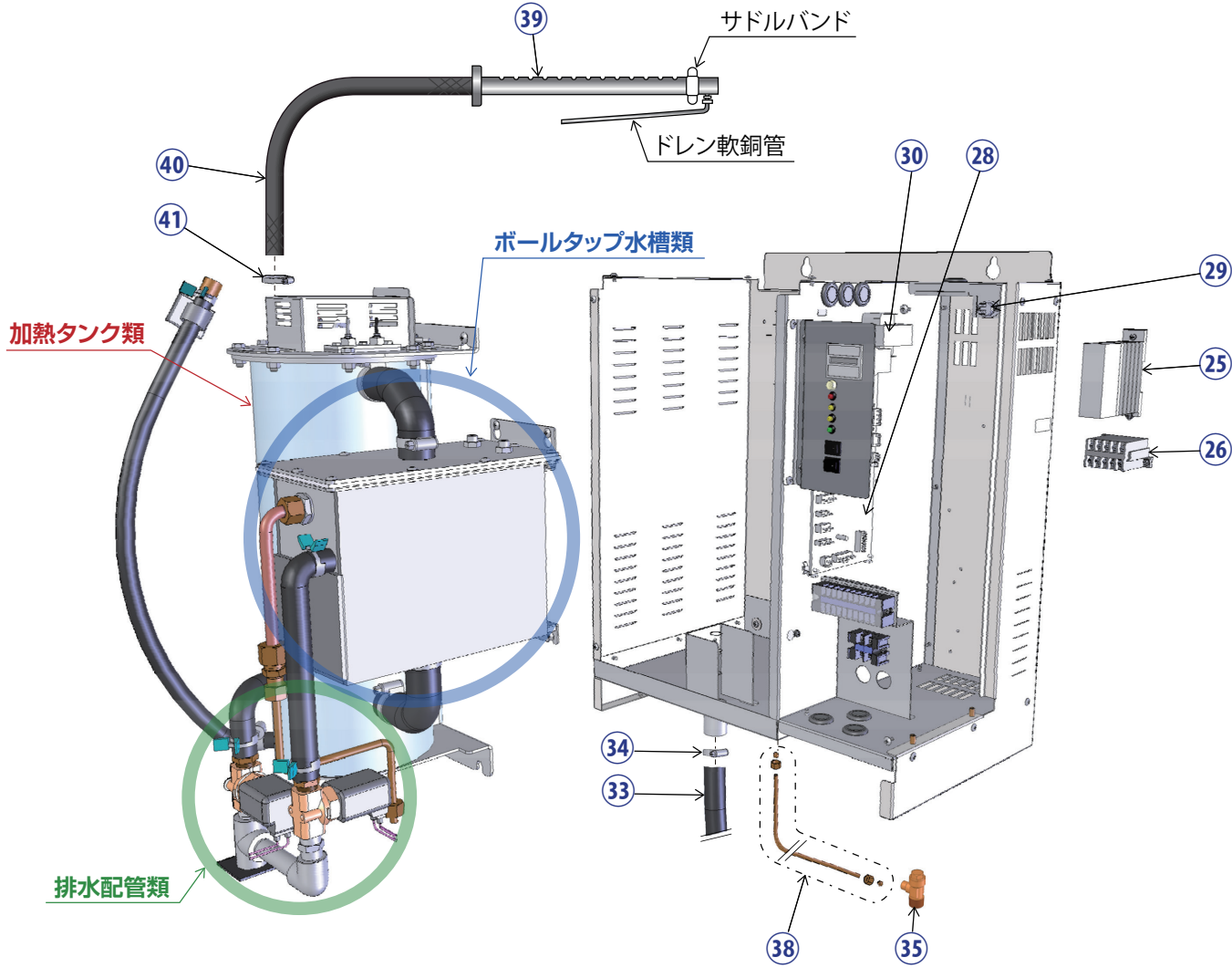
排水配管類
