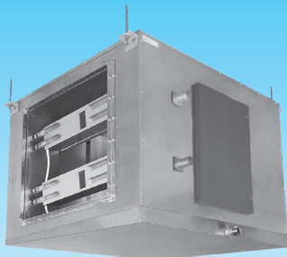
ダクト接続用加湿ユニット WM-SBA-Pシリーズ
