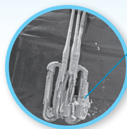
ヒータの周りに多量のスケールが析出している
