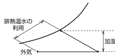
VRF/VHRタイプを利用した省エネシステムの場合
