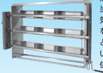
空調機組込用 WM-SBA-Hシリーズ
